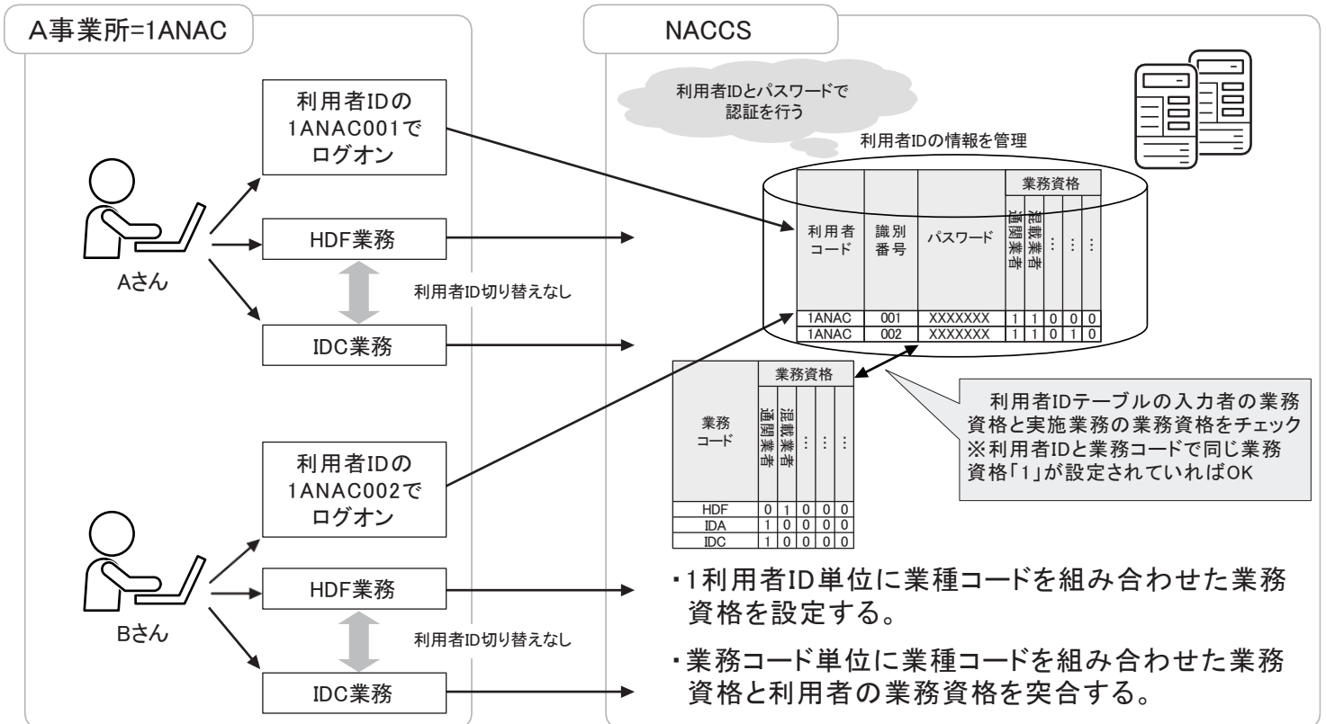
図7-2-1 複数業種を兼業する利用者の業務イメージ (シングルサインオンを使用した場合)
