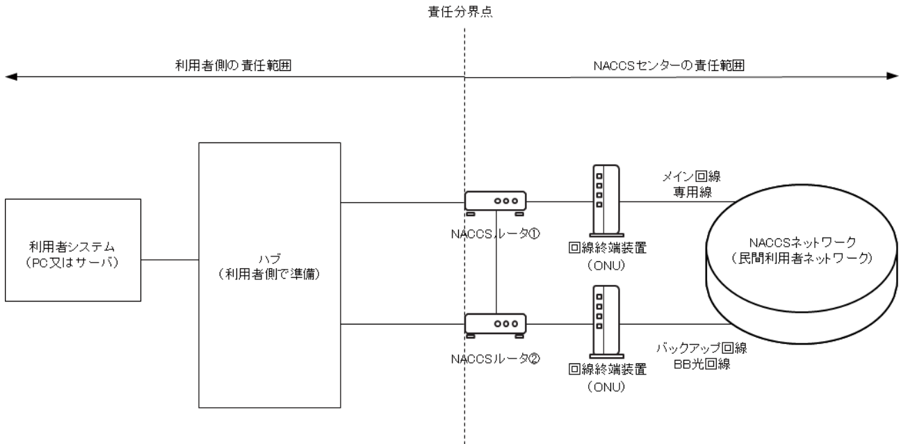
図 2-5-1 冗長化構成の概要
