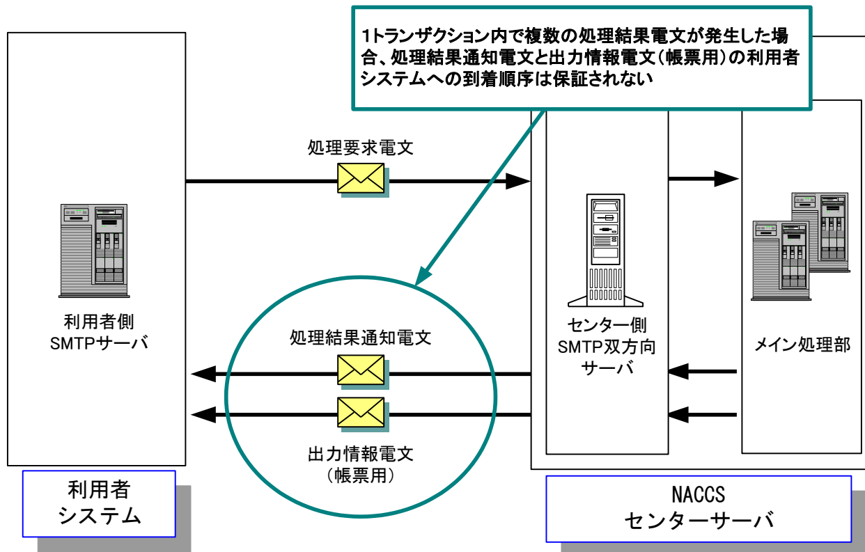
図 4-2-17 複数の処理結果電文の到着順序について (例)
