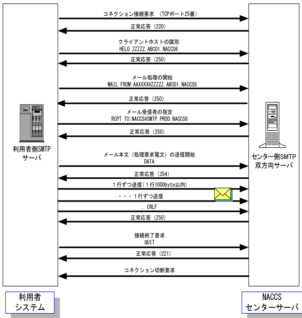
図 4-2-3 処理要求電文送信時の SMTP コマンドシーケンス
