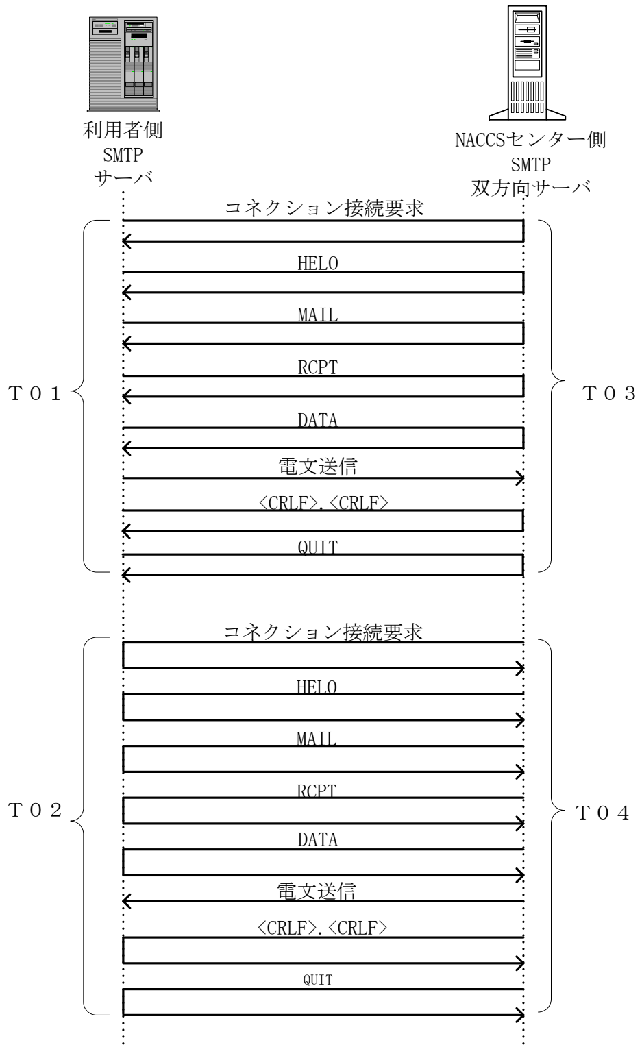
図 4-2-19 通常通信時のタイマー設定
