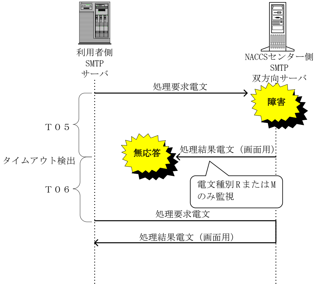
図 4-2-20 処理結果電文のタイマー監視
