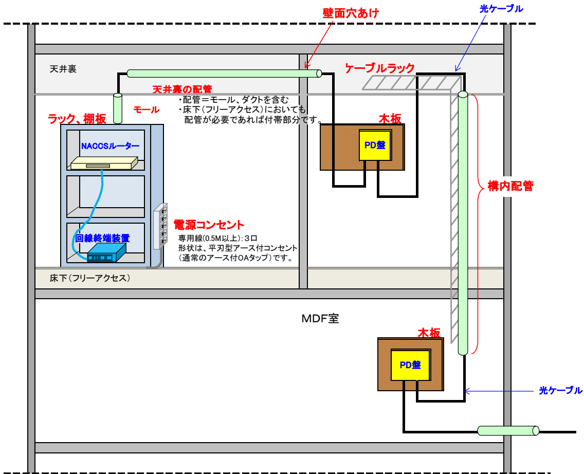
※図は、建物内光ケーブルルートの一例です
